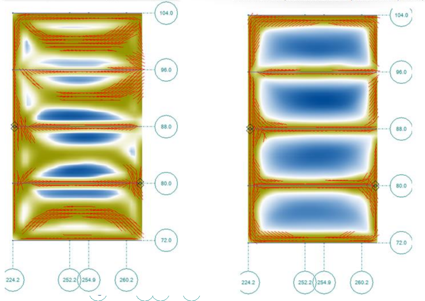
Главные напряжения \sigma_1 / 2-Средний Слой (тс/м 2 )
