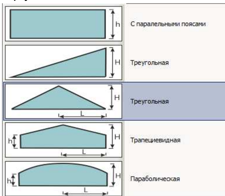
Рис. 3.20 Шаблоны ферм
