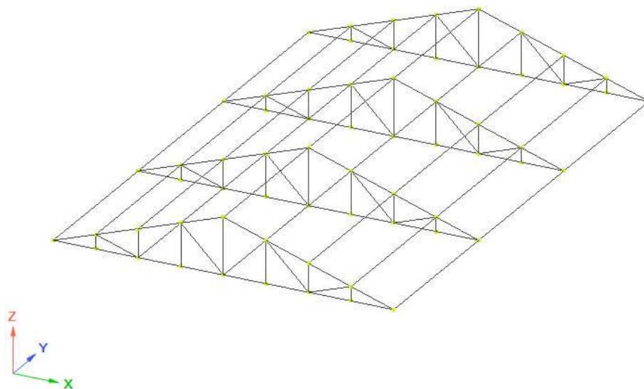
Рис. 3.27 Установка прогонов
