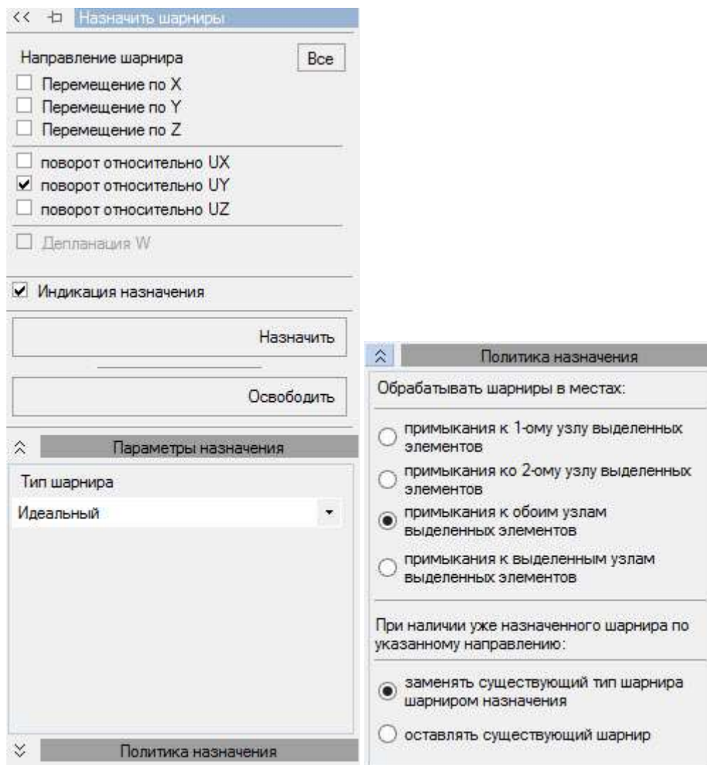
Рис. 3.30 Назначение шарниров
